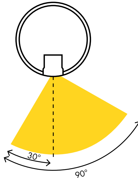
Asymmetrisk 90° Monteras vertikalt
