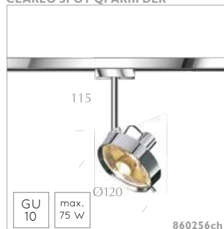
STAR CLAREO SPOT QPARIII DLR
