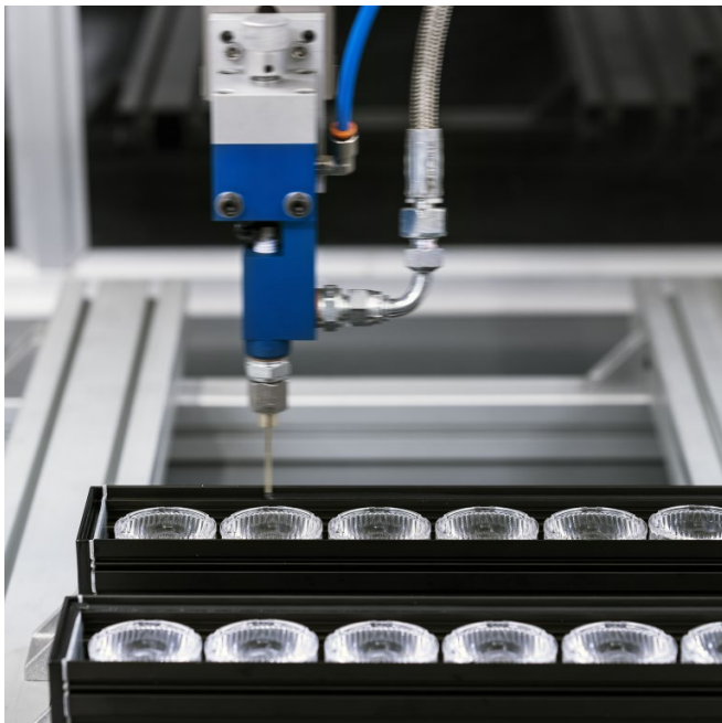
Siliconatura del diffusore Diffuser bonding machine
